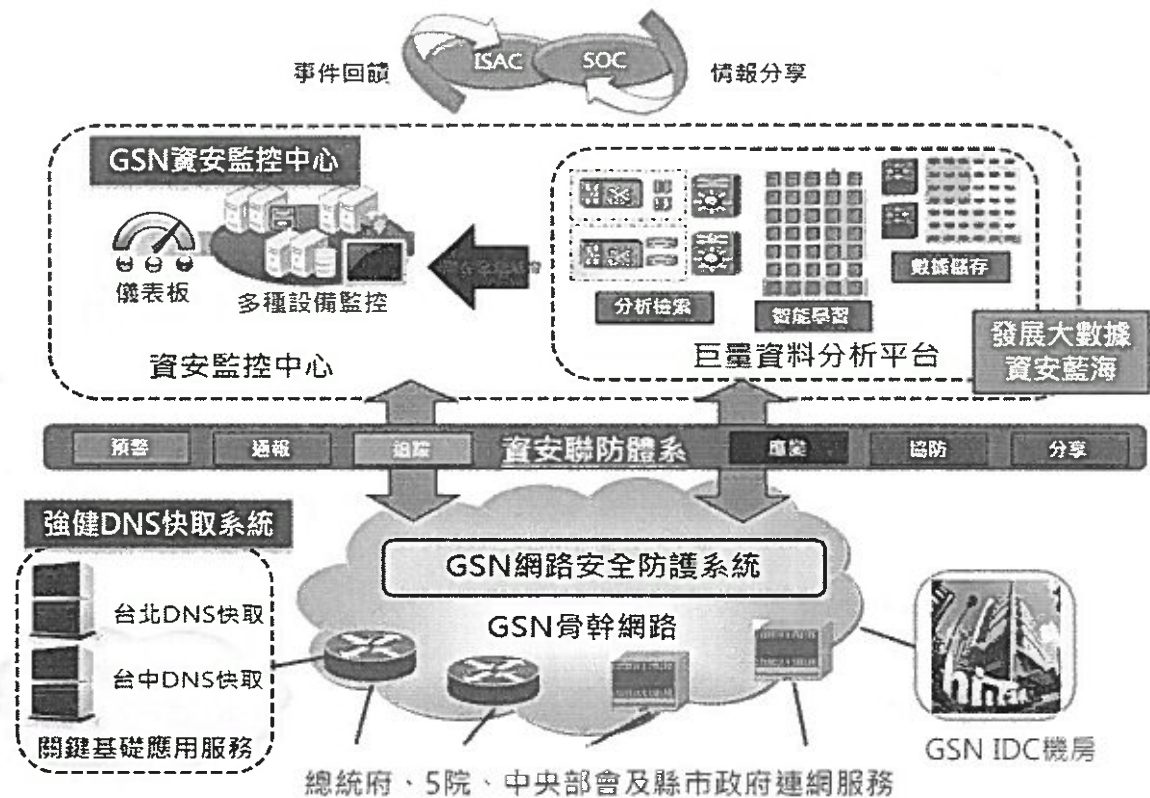
GSN 資安監控中心及巨量資料分析平台示意圖
